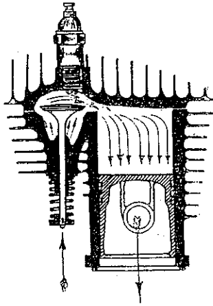
1 er TEMPS ( Admission )
