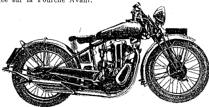
MOTOCYCLETTE 500 cm 3 CULBUTEURS, VUE DU COTÉ DISTRIBUTION
