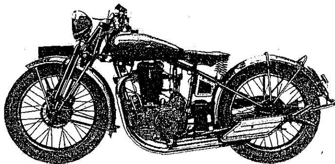
MOTOCYCLETTE 500cm 3 CULBUTEURS, VUE DU COTÉ EMBRAYAGE
