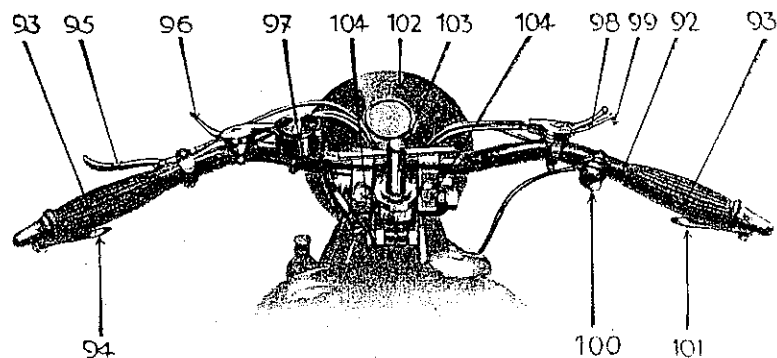
GUIDON AVEC LES POIGNÉES ET MANETTES DE COMMANDE
