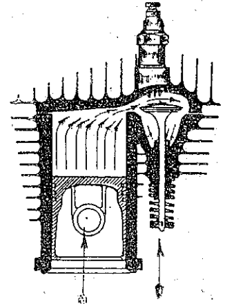
4 e TEMPS Echappement
