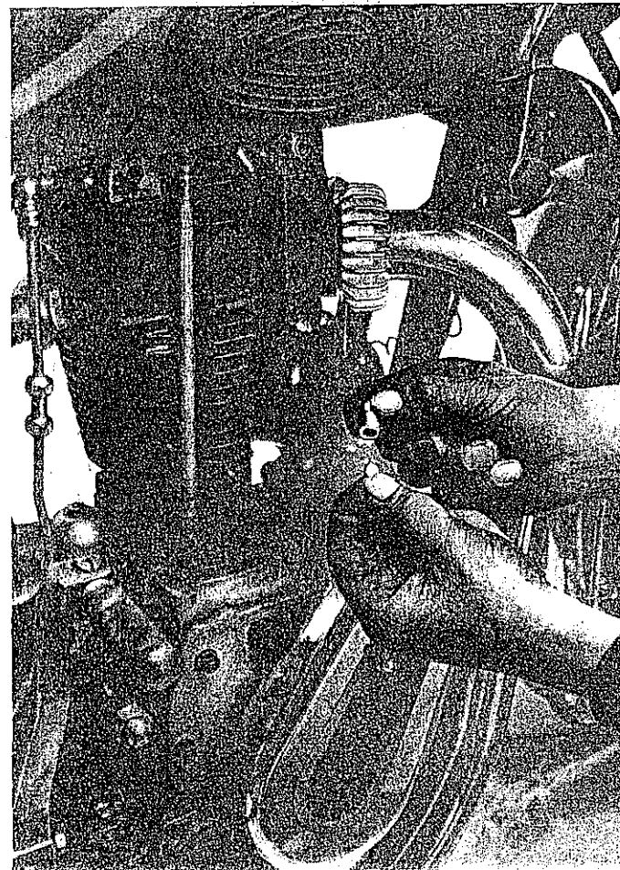
RÉGLAGE DU JEU DES SOUPAPES PAR CALES D'ÉPAISSEUR BLOC-MOTEUR A SOUPAPES LATÉRALES ET CULBUTEURS SPORT (Mise en place de la Cale d'épaisseur)
