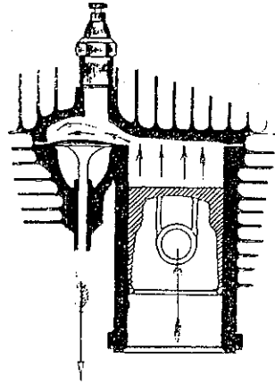
2 e TEMPS ( Compression )
