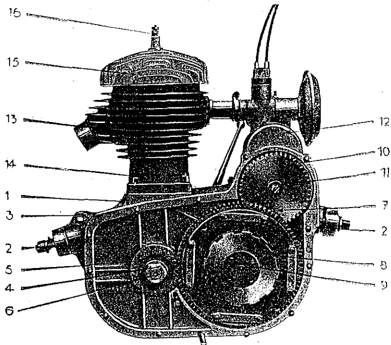
BLOC-MOTEUR A SOUPAPES LATÉRALES VU DU COTÉ GAUCHE (Le couvercle d'embrayage enlevé)
