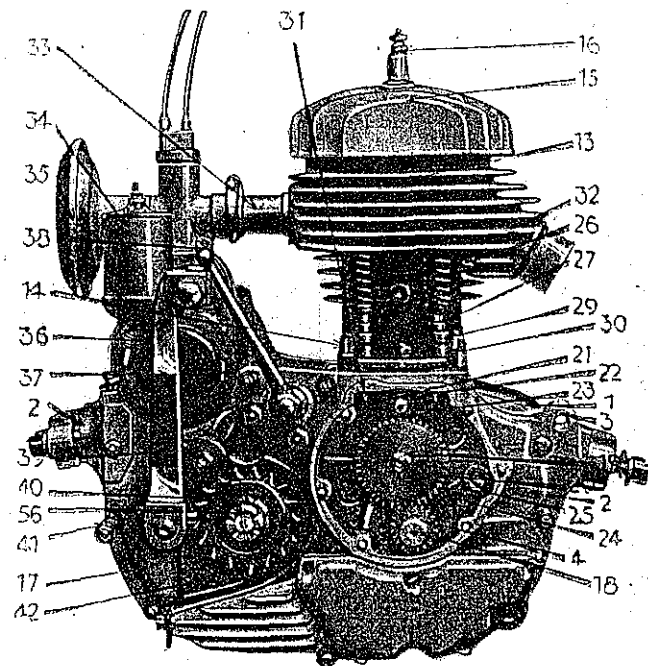
BLOC-MOTEUR A SOUPAPES LATÉRALES VU DU COTÉ DROIT (Le chapeau de distribution enlevé)
